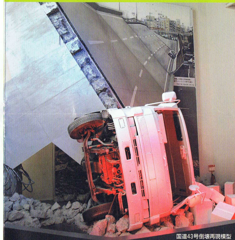
国道43号倒壊再現模型
